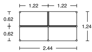
Módulo 4 usuarios con ducto cableable debajo de cubierta
